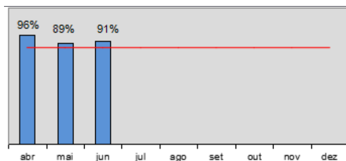
Percentual executado de Manutenção corretiva mensalmente
