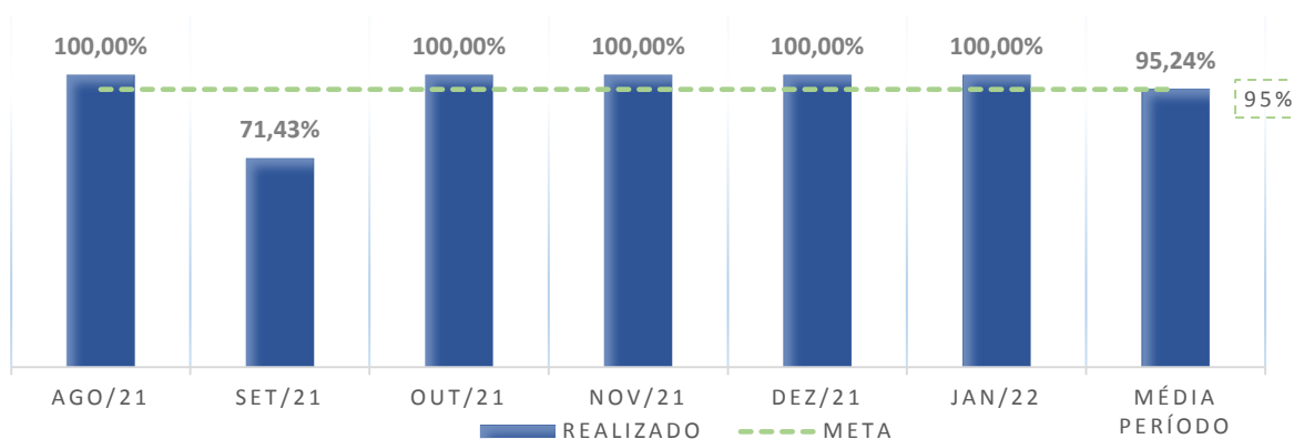
Gráfico 47 - Percentual de manutenções preventivas nos equipamentos realizadas na UCT - agosto de 2021 a janeiro de 2022
