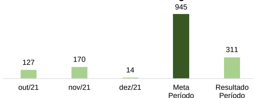
Gráfico nº 10 –Eletrocardiograma
