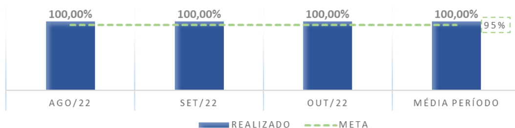
Gráfico 65 - Percentual de calibrações realizadas nos equipamentos da UCT - agosto a outubro de 2022
